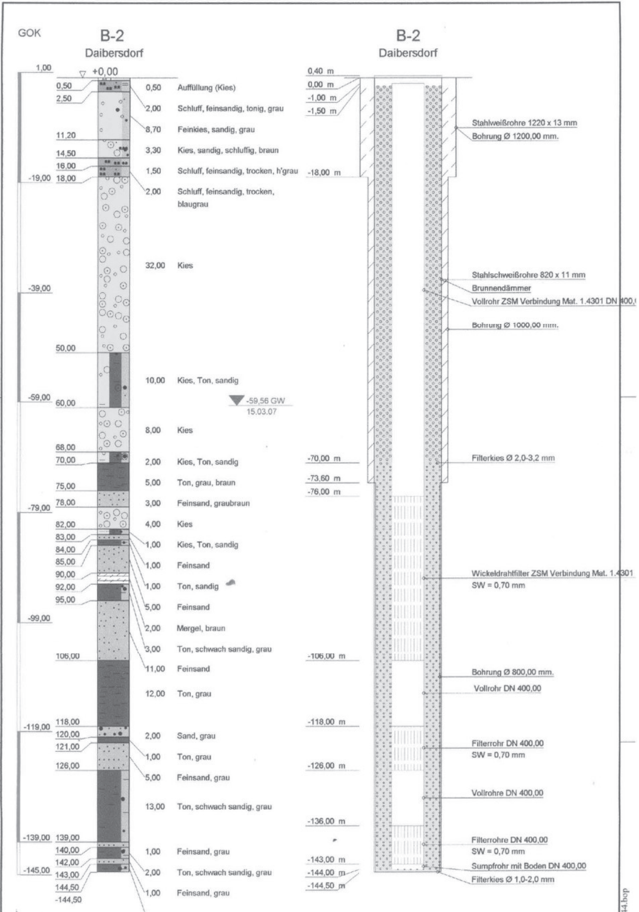
Ausbauplan Brunnen 2
